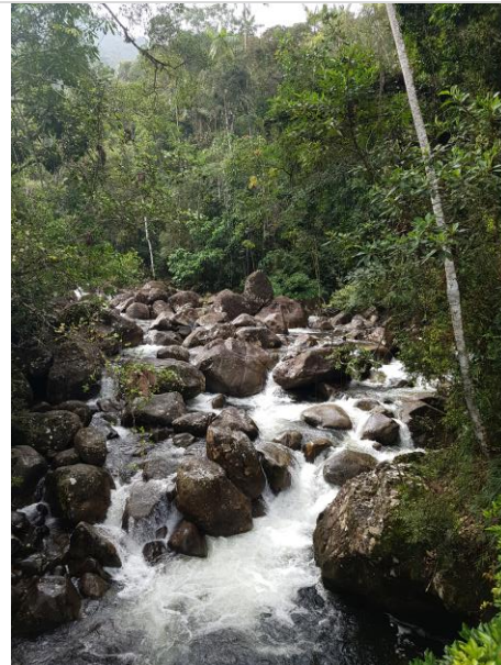
Figura 8 – Detalhe de trecho do rio Campo Belo, a montante do Lago Azul, PNI.
